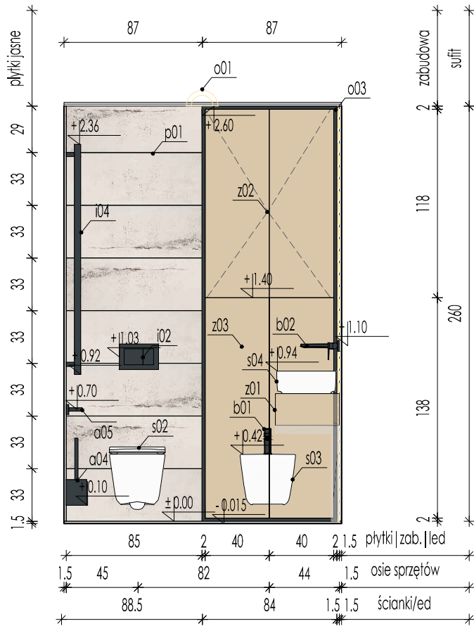
WIDOK D-D
