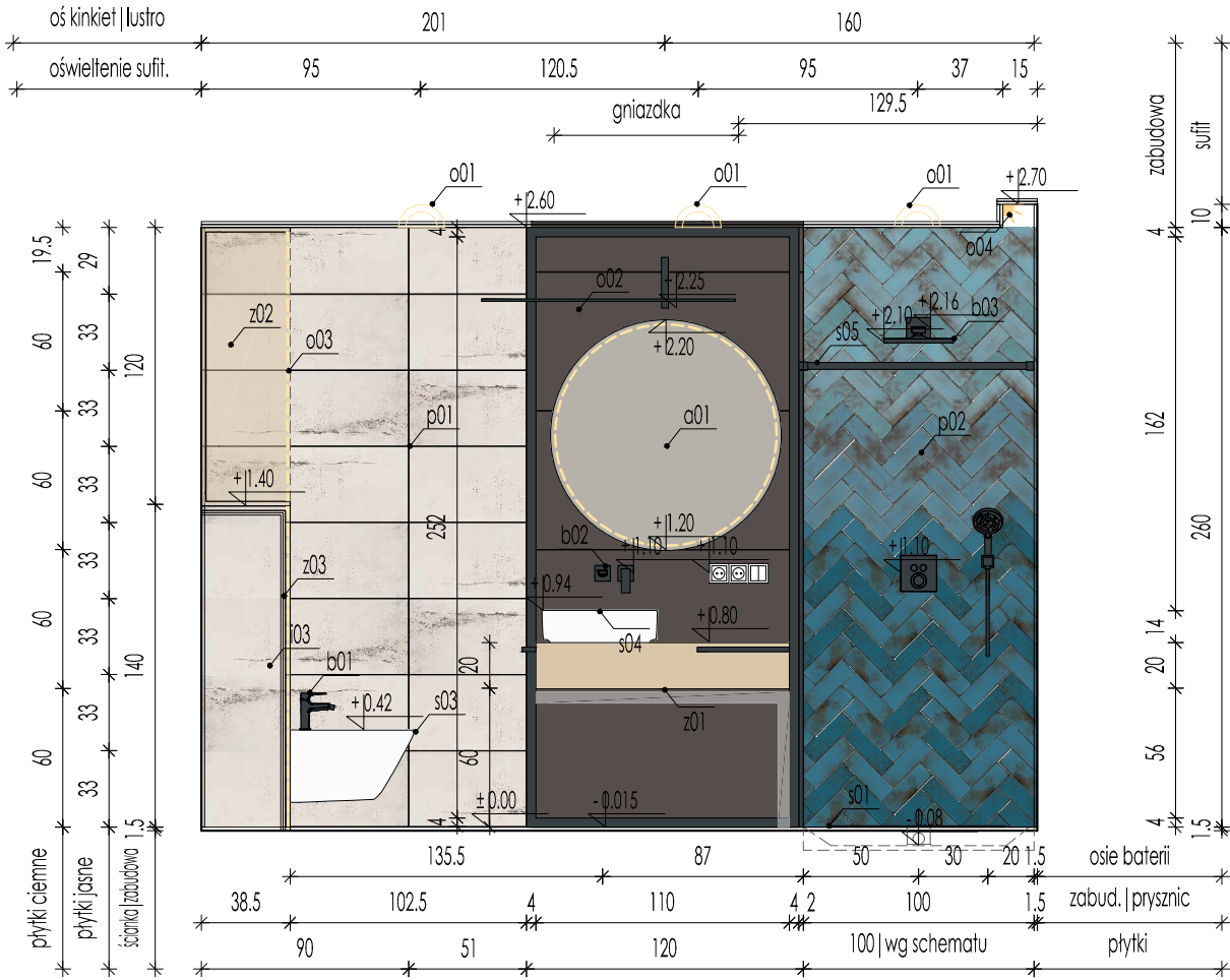
WIDOK A-A
